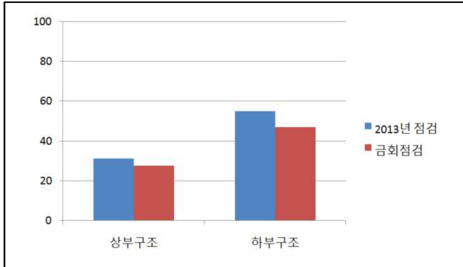
【그림 4.4】 부재별 탄산화깊이에 의한 콘크리트 잔여피복두께 비교
